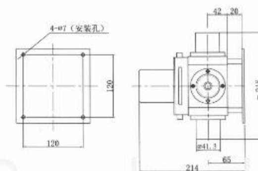
外形图
